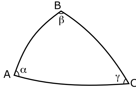
Рис. 2: Пояснение смысла геометрических параметров однородных эйнштейновских вакуумов; AB, BC, AC - геодезические. \Sigma = \alpha + \beta + \gamma ; S - площадь треугольника ABC . Кривизна R_3 по определению: R_3 = (\Sigma - \pi)/S = 3k/a^2 , a - радиус кривизны. При k = 0 , \Sigma = \pi ; k = +1 , \Sigma > \pi ; k = -1 , \Sigma < \pi .
